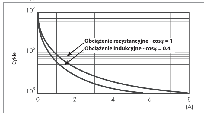
F 40.4 - Trwałość łączeniowa (dla AC) w funkcji prądu na zestykach Typ 40.52 (strona 4)
