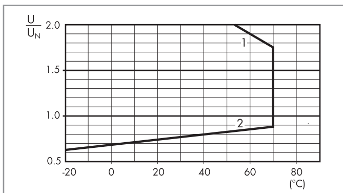
R 40 - DC Dopuszczalny zakres napięcia pracy cewki w zależności od temperatury otoczenia - Wykonanie czułe, typ 40.11
