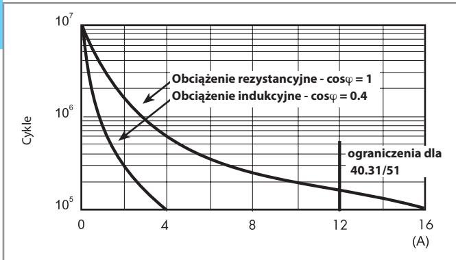
F 40.3 - Trwałość łączeniowa (dla AC) w funkcji prądu na zestykach Typ 40.31/51/61 (strona 4)
