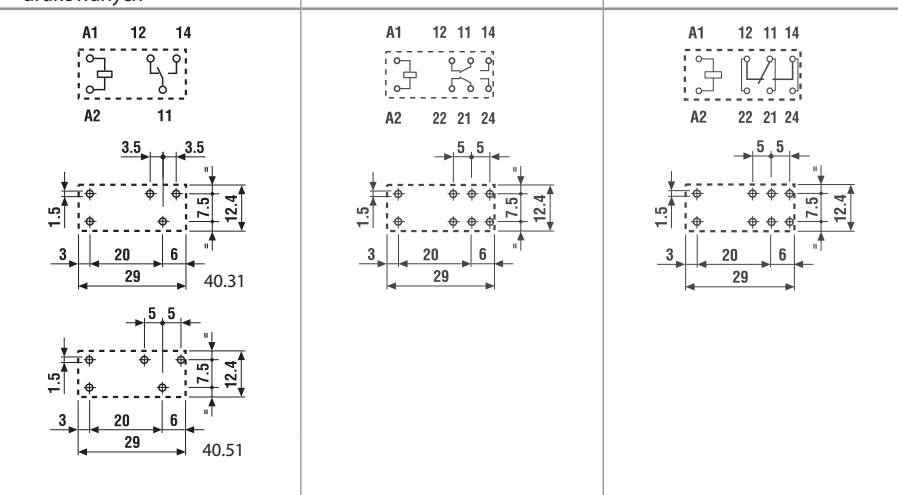
Rysunek otworów montażowych Długość pinów 5.3 mm dla gniazd i obwodów drukowanych
