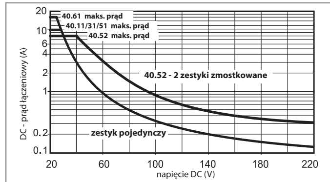
H 40.2 - Obciążenie graniczne dla prądu stałego (dla DC1) Typ 40.31/51/52/61 (strona 4) i 40.11 (strona 5)
