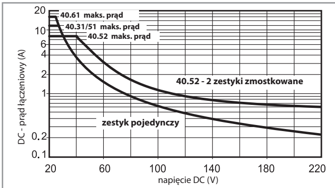
H 40.1 - Obciążenie graniczne dla prądu stałego (dla DC1) Typ 40.31/51/52/61 (strona 3)
