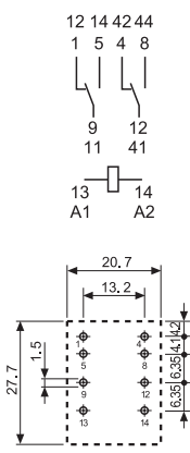
Rysunek otworów montażowych
