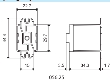
Adapter tylny do mocowania na obudowie dla 55.32, 55.33, 55.34
