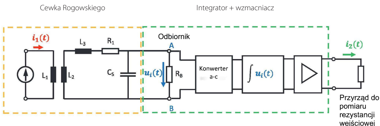
Rys. 3: Elektryczny obwód zastępczy cewki Rogowskiego z integratorem 1 A
