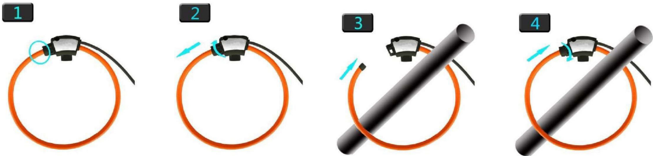
Rys. 6: Montaż cewki FASK
