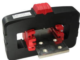
Przekładniki do ferm wiatrowych
