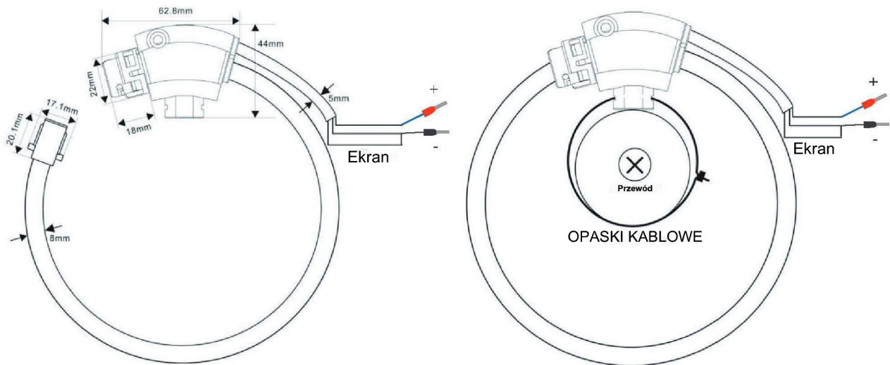
Rys. 7: Inne wymiary FAK 100, 150, 200 i 300
