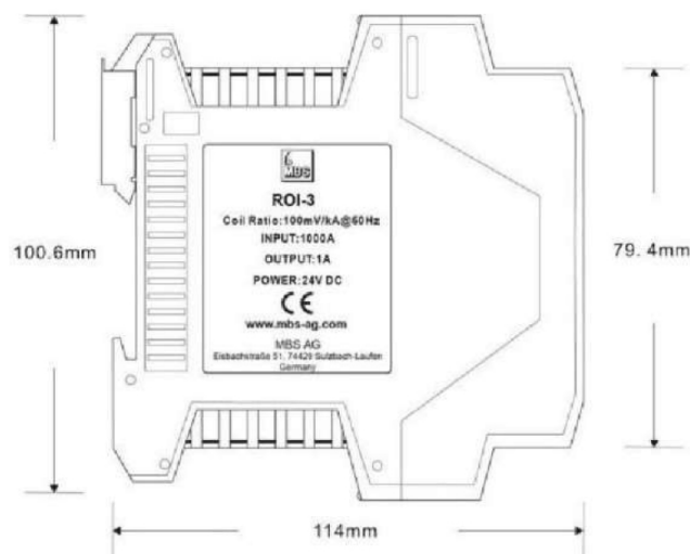
Rys. 9: Wymiary ROI-3
