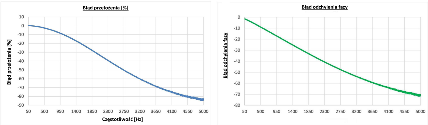
Rys. 11: Charakterystyka przenoszenia częstotliwości przez ROI-3 z cewką Rogowskiego FASK 150 (błąd amplitudy i odchylenia fazy)
