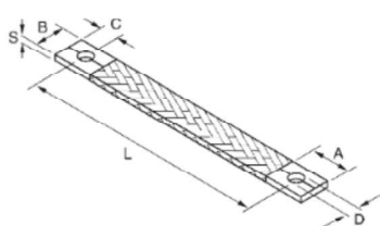
Złącze standardowe D / Standard terminal D
