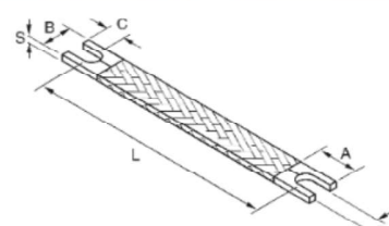
Złącze widelkowe F / Fork terminal F
