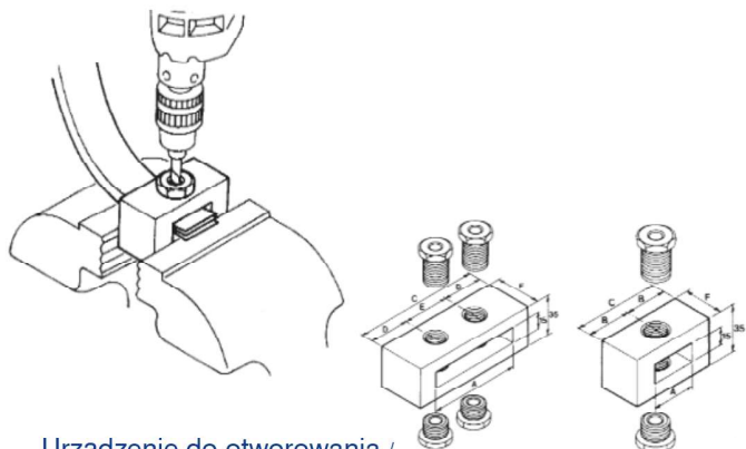
Urządzenie do otworowania / Drilling devices
