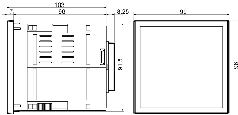
Agujero/ Panel hole: 91,5 x 91,5 mm
