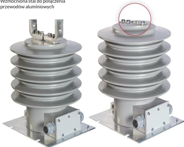
Wzmocniona stal do połączenia przewodów aluminiowych
