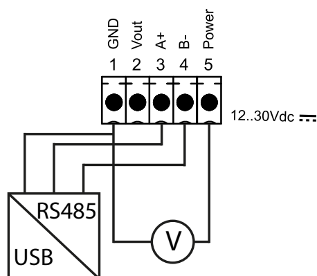
Anschlussschema BT7000
