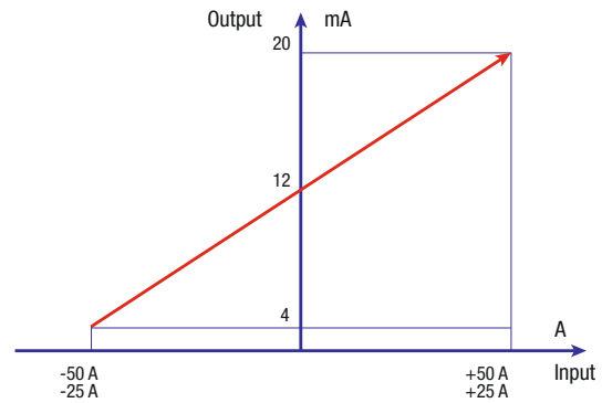
Input / Output
