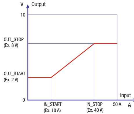
Input / Output
