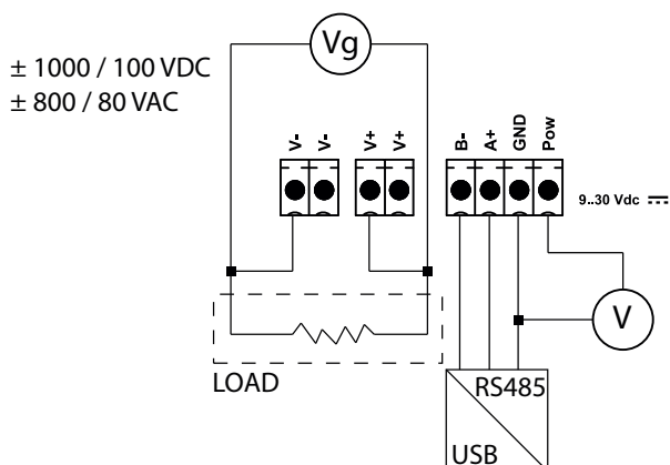
Anschlusschema BT7300 / BT7350
