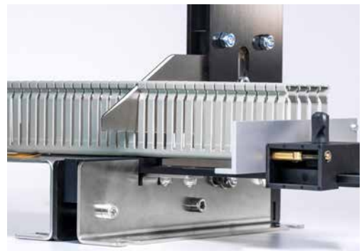
Messerschutz/Blade protection
