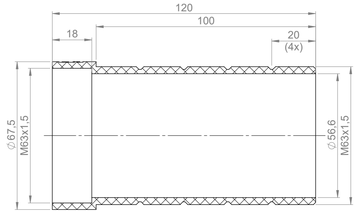
SCHNITT A-A
