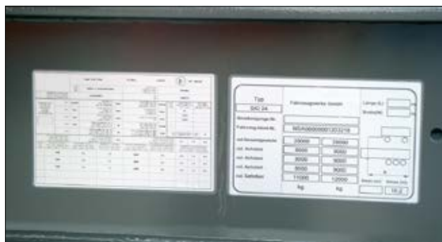
Tabliczka znamionowa naczepy samochodowej zabezpieczona laminatem.
