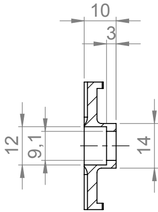
SCHNITT A-A
