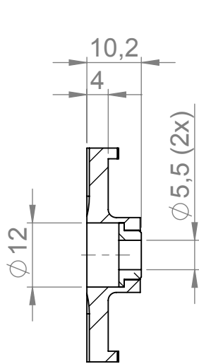
SCHNITT A-A
