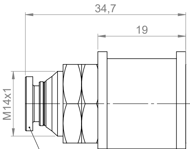
Schottkupplung für Pneumatikschlauch Ø6mm (Bulkhead coupling for pneumatic pipe Ø6mm)
