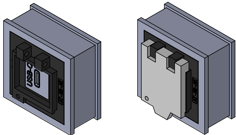
Darstellung ohne Abdeckkappe shown without cover cap
