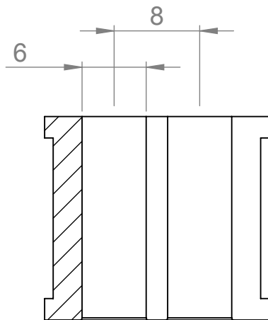
SCHNITT A-A
