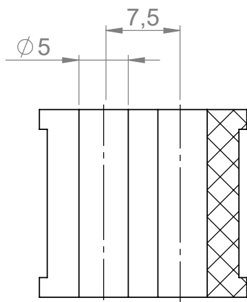
SCHNITT A-A
