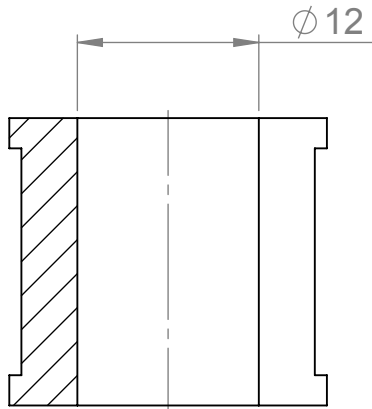
SCHNITT A-A
