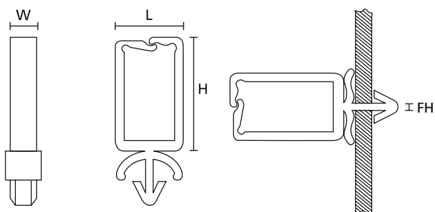
WPC (widok z boku, widok z góry, w zastosowaniu)
