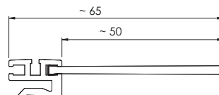
długość samej szczotki 50 mm
