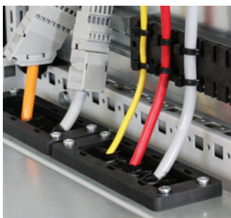
Dopasowany do konstrukcji szafy sterowniczej...
