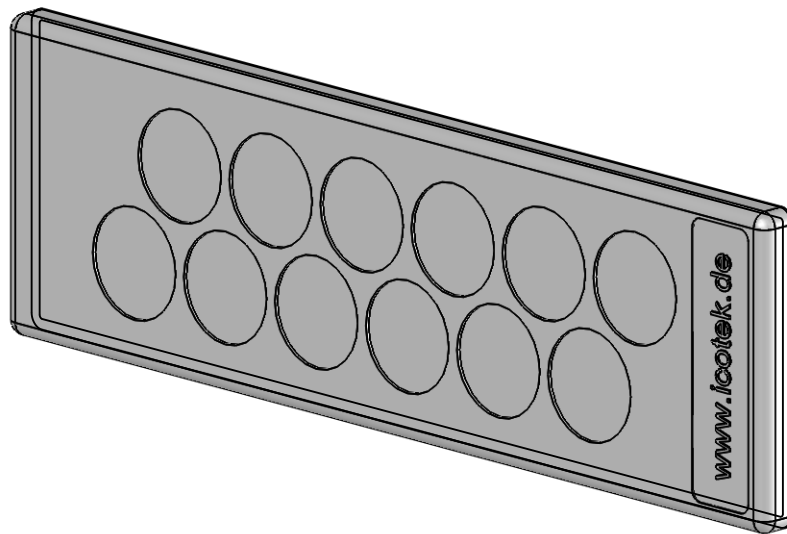
Kabeldurchführungsplatte KEL-DP 24/12 A 12 x Ø 15 mm für Blechstärken von 1,5 - 2,5 mm
