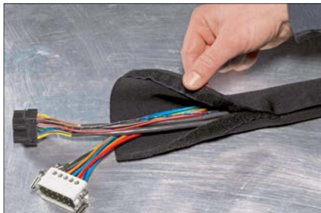
Osłona ochronna HELAHOOK umożliwia rozpięcie i ponowne użycie.
