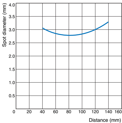
E3Z-L□1(L□6)
