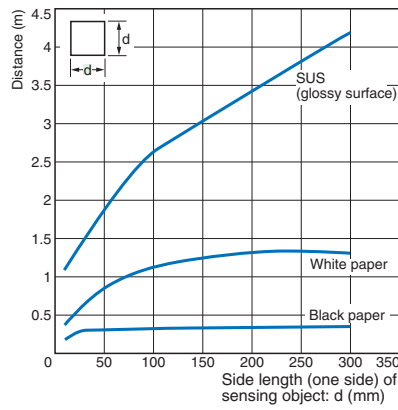
E3Z-D□2(D□7)
