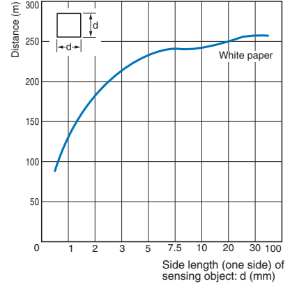
E3Z-L□1(L□6)
