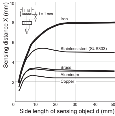
E2A-S12□N08
