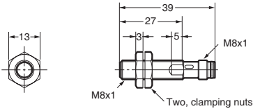
E2A-S08KS02-M5-□□/ E2A-S08KS02-M3-□
