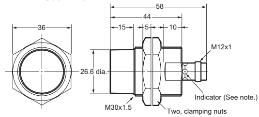
E2A-S30KN20-M1-□
