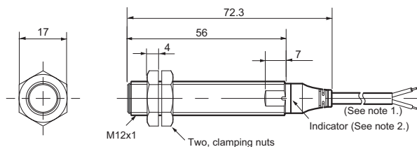
E2A-S12LS04-WP-□
