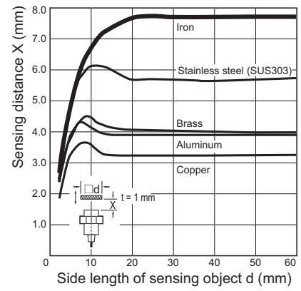
E2A-S18 □ S08
