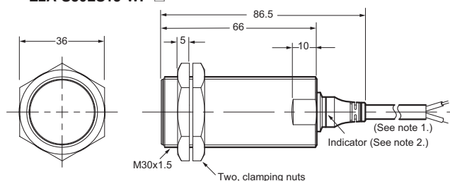
E2A-S30LS15-WP-□
