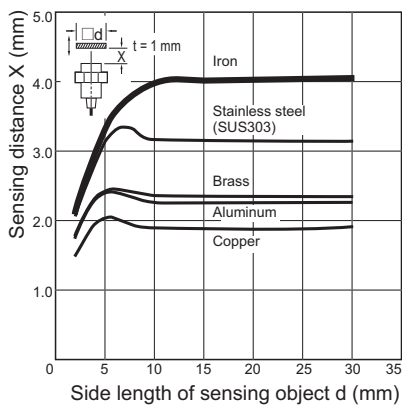
E2A-S12 □ S04
