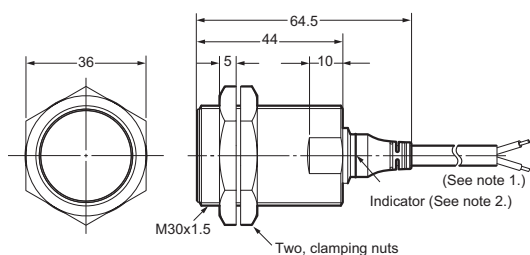
E2A-S30KS15-WP-□
