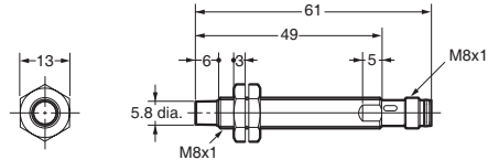
E2A-S08LN04-M5-□□/ E2A-S08LN04-M3-□
