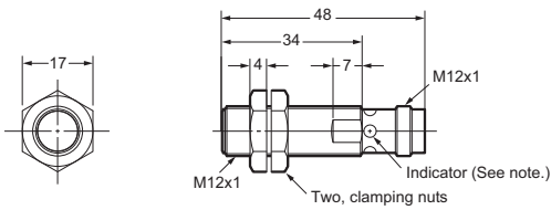
E2A-S12KS04-M1-□
