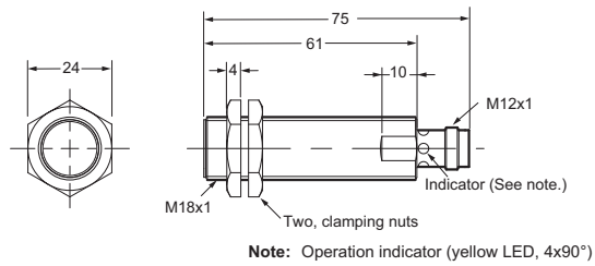
E2A-S18LS08-M1-□
