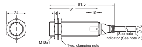
E2A-S18LS08-WP-□
