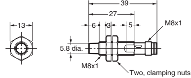
E2A-S08KN04-M5-□□/ E2A-S08KN04-M3-□
