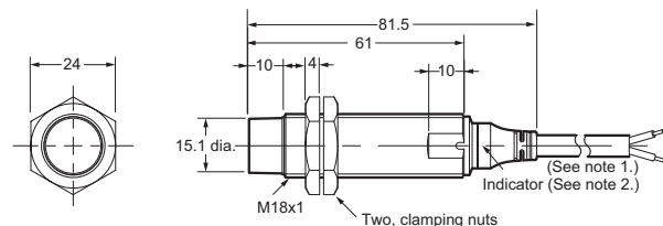
E2A-S18LN16-WP-□
