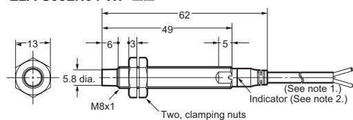
E2A-S08LN04-WP-□□
