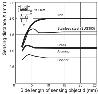
E2A-S30 □ S15
