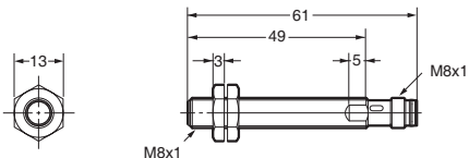
E2A-S08LS02-M5-□□/ E2A-S08LS02-M3-□
