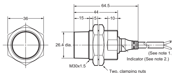
E2A-S30KN20-WP-□
