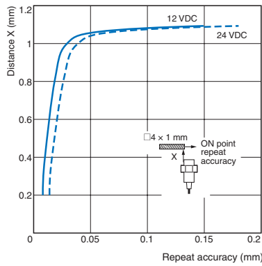
E2E-C04S12□/E2E-S05S12□
