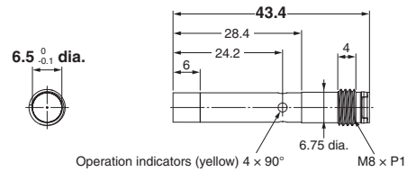
E2E-C06N04-MC-□□
