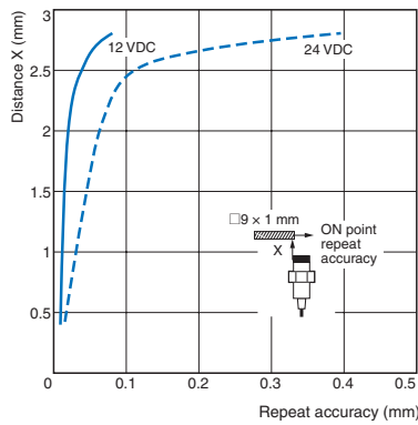
E2E-C04N03□/E2E-S05N03□
