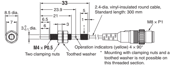
E2E-S04N02-CJ-□□
