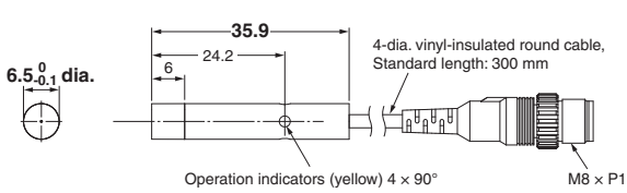
E2E-C06N04-CJ-□□
