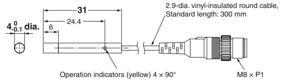
E2E-S04N02-CJ-□□
