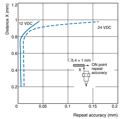
E2E-C05S01□
