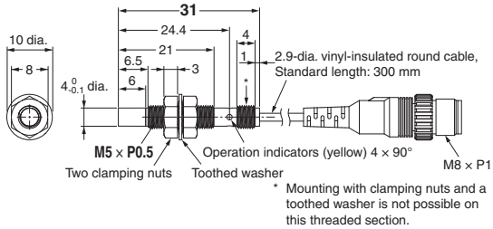
E2E-S05N03-CJ-□□
