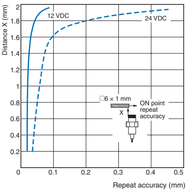
E2E-C03N02□/E2E-S04N02□
