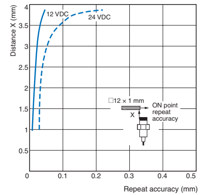
E2E-C06N04□
