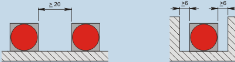
Type SIP17
