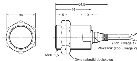
E2A-M30KS15-WP-□□/E2A-S30KS15-WP-□
