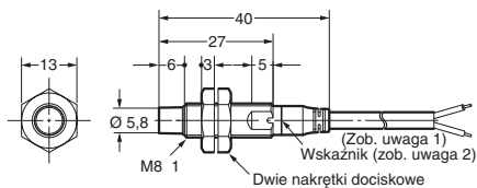
E2A-S08KN04-WP-□□
