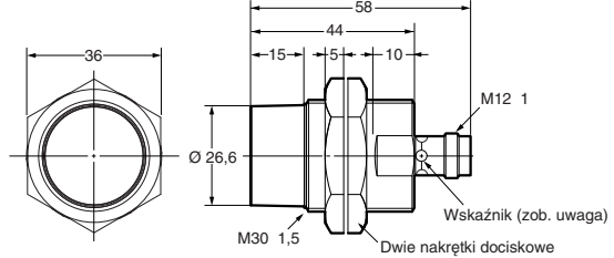
E2A-M30KN20-M1-□□/E2A-S30KN20-M1-□
