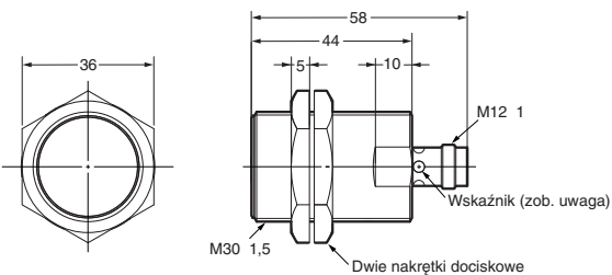
E2A-M30KS15-M1-□□/E2A-S30KS15-M1-□
