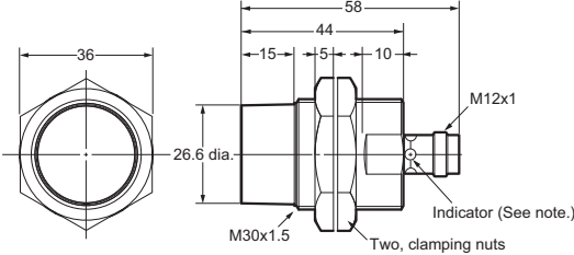
E2A-S30KN20-M1-□
