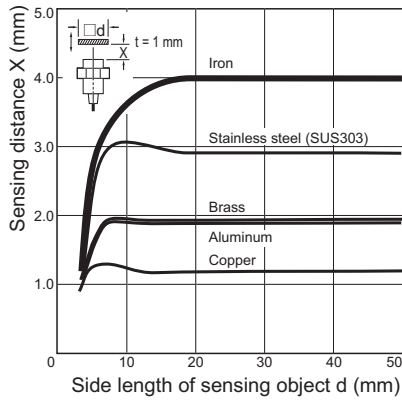
E2A-S08□N04
