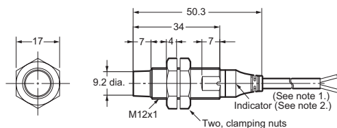
E2A-S12KN08-WP-
