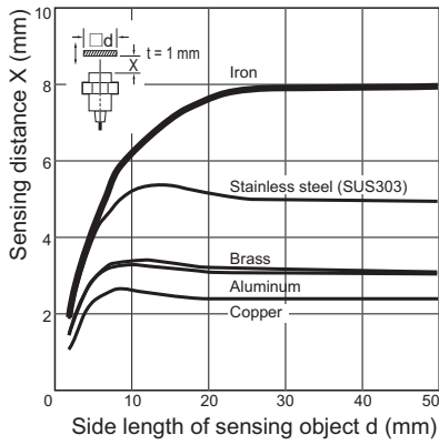
E2A-S12□N08
