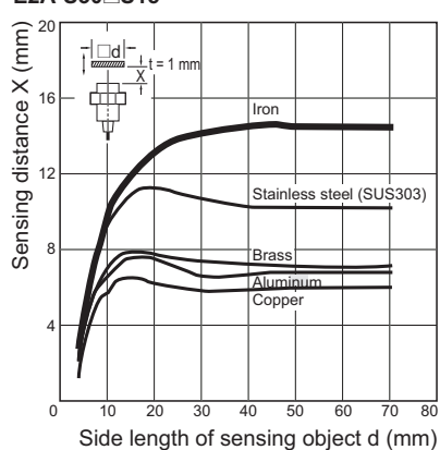
E2A-S30□S15
