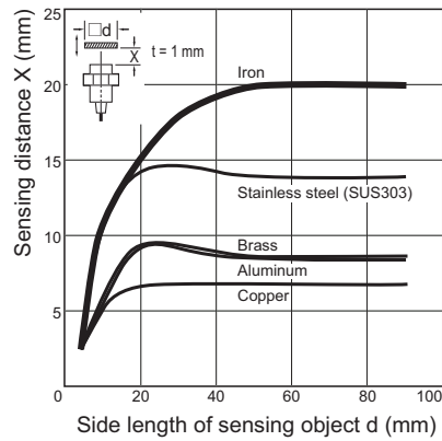
E2A-S30KN20
