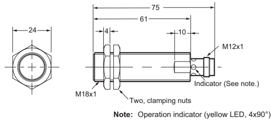
E2A-S18LS08-M1-□
