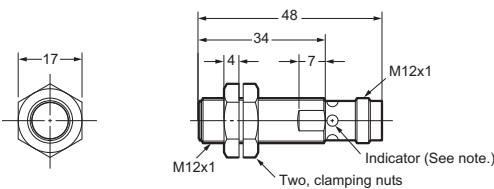
E2A-S12KS04-M1-□
