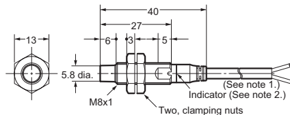
E2A-S08KN04-WP-□□
