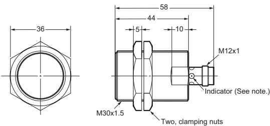
E2A-S30KS15-M1-□
