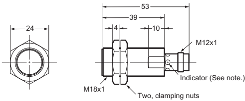
E2A-S18KS08-M1-□
