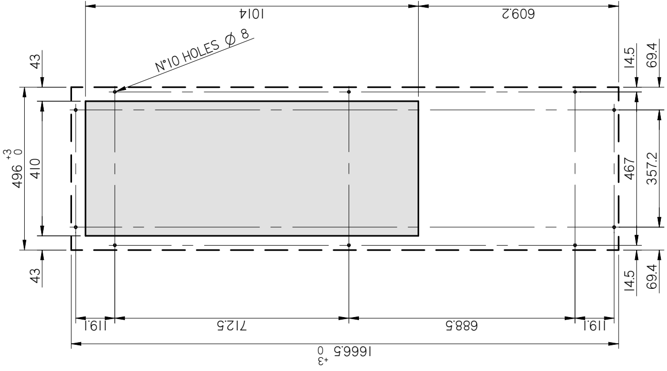
MONTAGGIO ESTERNO EXTERNAL MOUNTING
