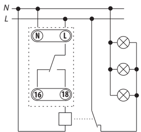
Bezpośrednie podłączenie oświetlenia awaryjnego (dla I < 16A)
