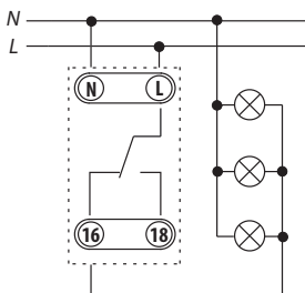
Podłączenie oświetlenia awaryjnego poprzez stycznik (dla I > 16A)
