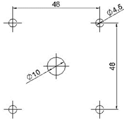
Bohrbild D1 (E) Drilling pattern D1 (E)
