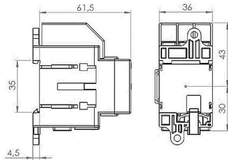
Grundkörper LO mit Bodenbefestigung (V) Base body LO with floor mounting (V)
