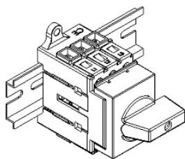
Bodenbefestigung (V) Floor mounting (V)
