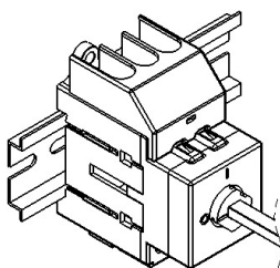
Zentrallochbefestigung (ZM) Central hole mounting (ZM)
