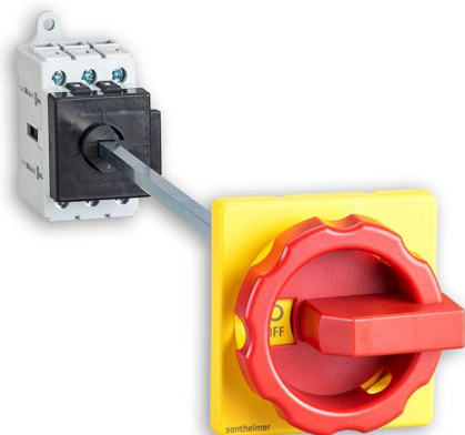
NLO Schalter mit Türkupplung Befestigungsart Bodenbefestigung V / NLO switch with door coupling Mounting type Floor mounting V
