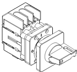
Vierlochbefestigung (E) Four-hole mounting (E)
