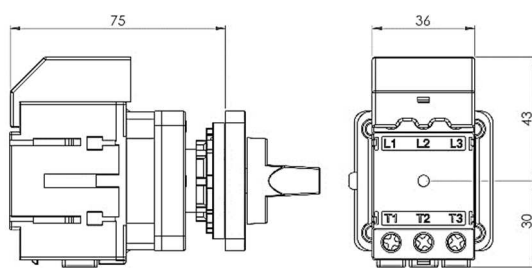
Grundkörper LO mit Zentrallochbefestigung (ZM) Base body LO with central hole mounting (ZM)
