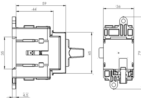
Grundkörper LO mit DIN-Normbefestigung (T) Base body LO with DIN standard mounting (T)
