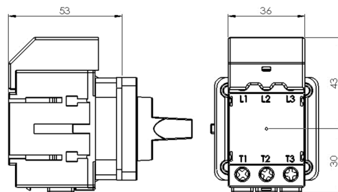
Grundkörper LO mit Vierlochbefestigung (E) Base body LO with four-hole fixing (E)
