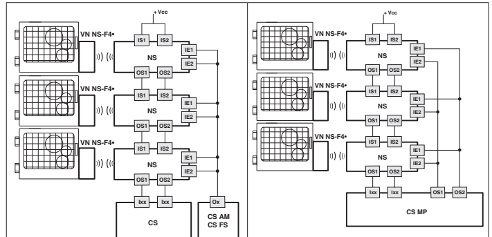
Fonction de surveillance de l'actionneur verrouillé : 2 canaux / catégorie 4 / jusqu'à SIL 3 / PL e
