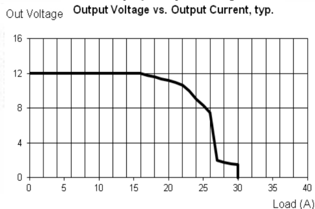
Zależność napięcia wyjściowego od prądu wyjściowego
