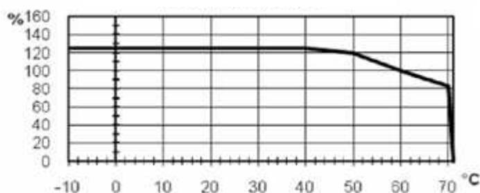
Krzywa spadku prądu wyjściowego zależnie od temperatury
