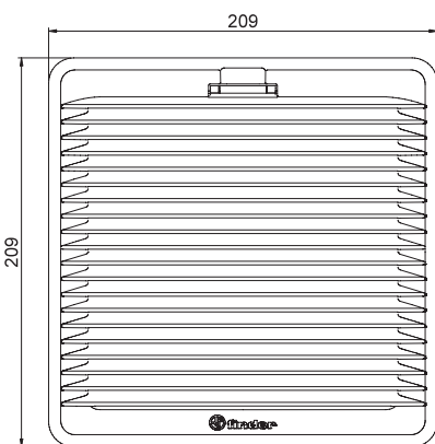
Type 7F.20.x.xxx.3100
