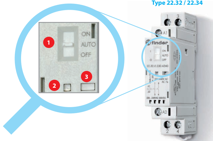
Type 22.32 / 22.34
