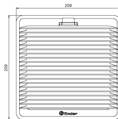
Type 7F.02.0.000.3000
