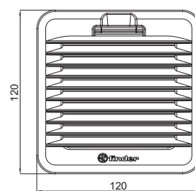
Type 7F.02.0.000.1000
