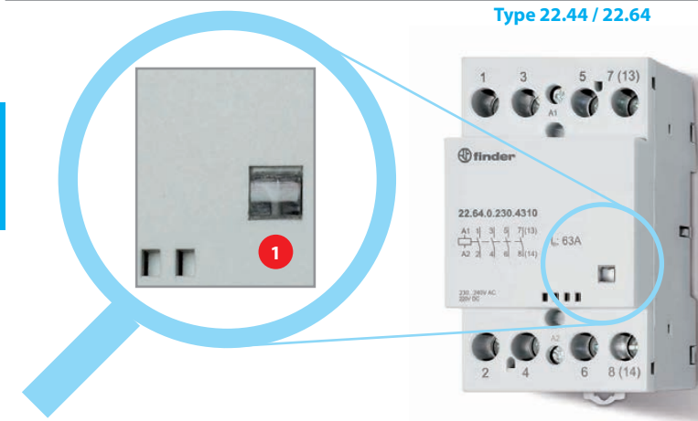
Type 22.44 / 22.64
