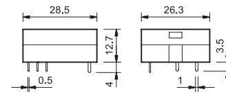
Type 40.11 (page 41)
