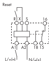
Schemat połączeń (Zasilany START)
