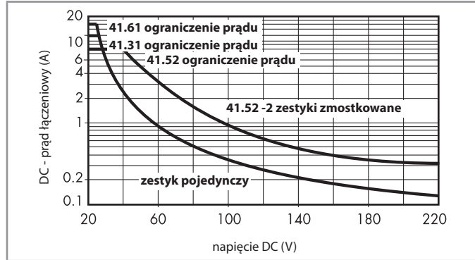
H 41 - Obciążenia graniczne dla prądu stałego (dla DC1)
