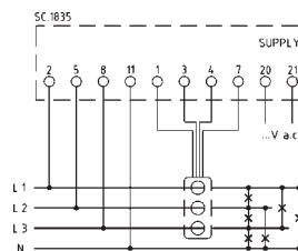
Q52D3L063X4C2 - Q52D3L125X4C2 system 3 fazowy, 4 przewodowy for three-phase four wires system
