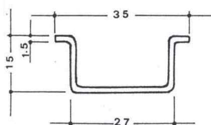
TS35/15 - wysoka
