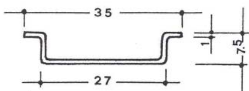
TS35/7,5 - niska
