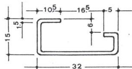
TS32/15 - profil G
