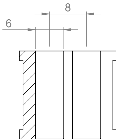
SCHNITT A-A
