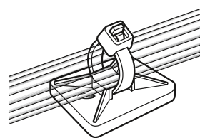
Zastosowanie cokołu MB3A
