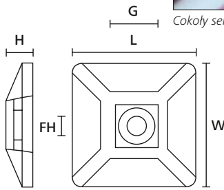
Cokół MB4CA (widok z boku i z góry)
