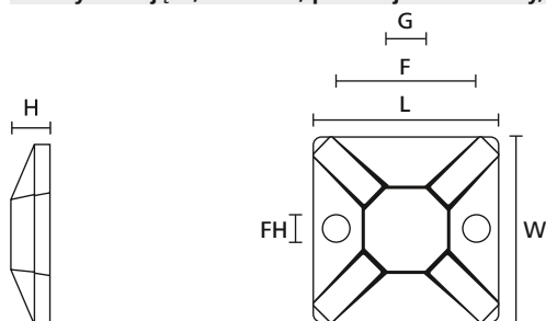
MB3-MB5 (widok z boku)
