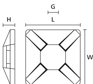
Cokół MB2A (widok z boku i z góry)
