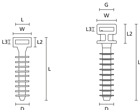
Kołek LOK01, LOK01B, LOK01S
