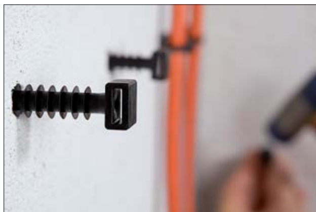
Kołki LOK01 do zastosowania wewnątrz i na zewnątrz.
