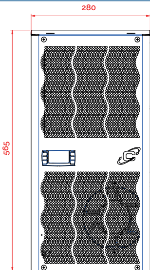
CNE07- 230V CNE07- 115V
