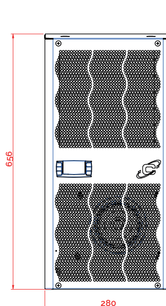
CNE04- 400V CNE04- 460V
