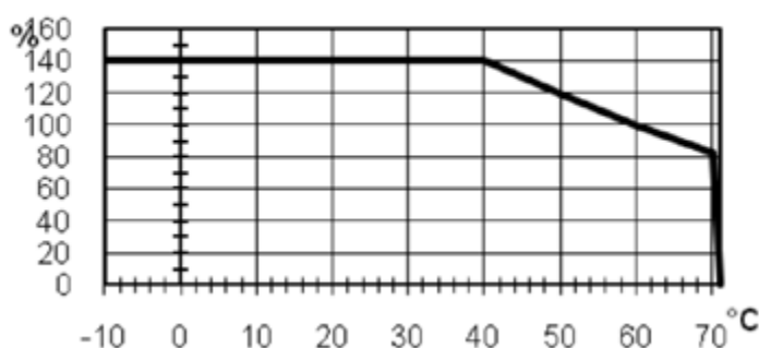
Krzywa spadku prądu wyjściowego zależnie od temperatury
